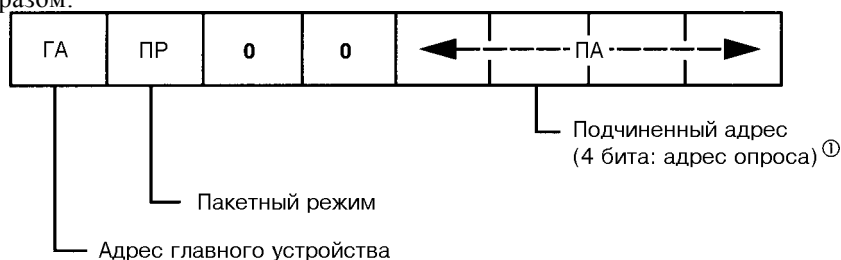
РИСУНОК 3-3. Адрес: Формат короткого фрейма.
