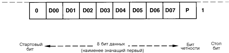
РИСУНОК 3-1. Последовательная передача одного 8-разрядного байта.
